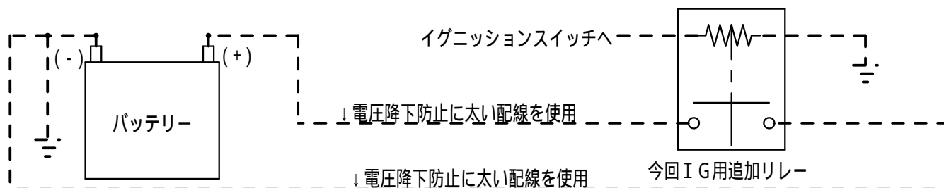
今回C.D.I.配線
