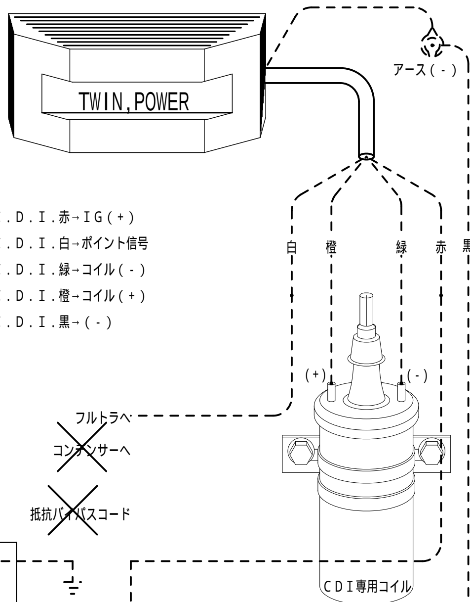
今回C.D.I.配線
